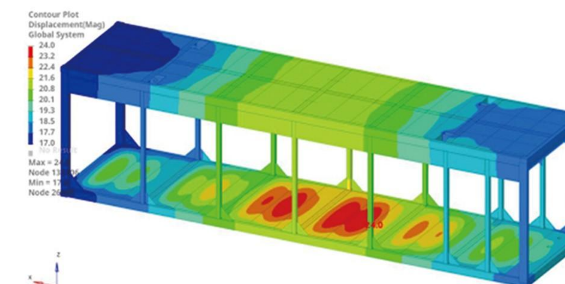
四点吊整体变形云图
