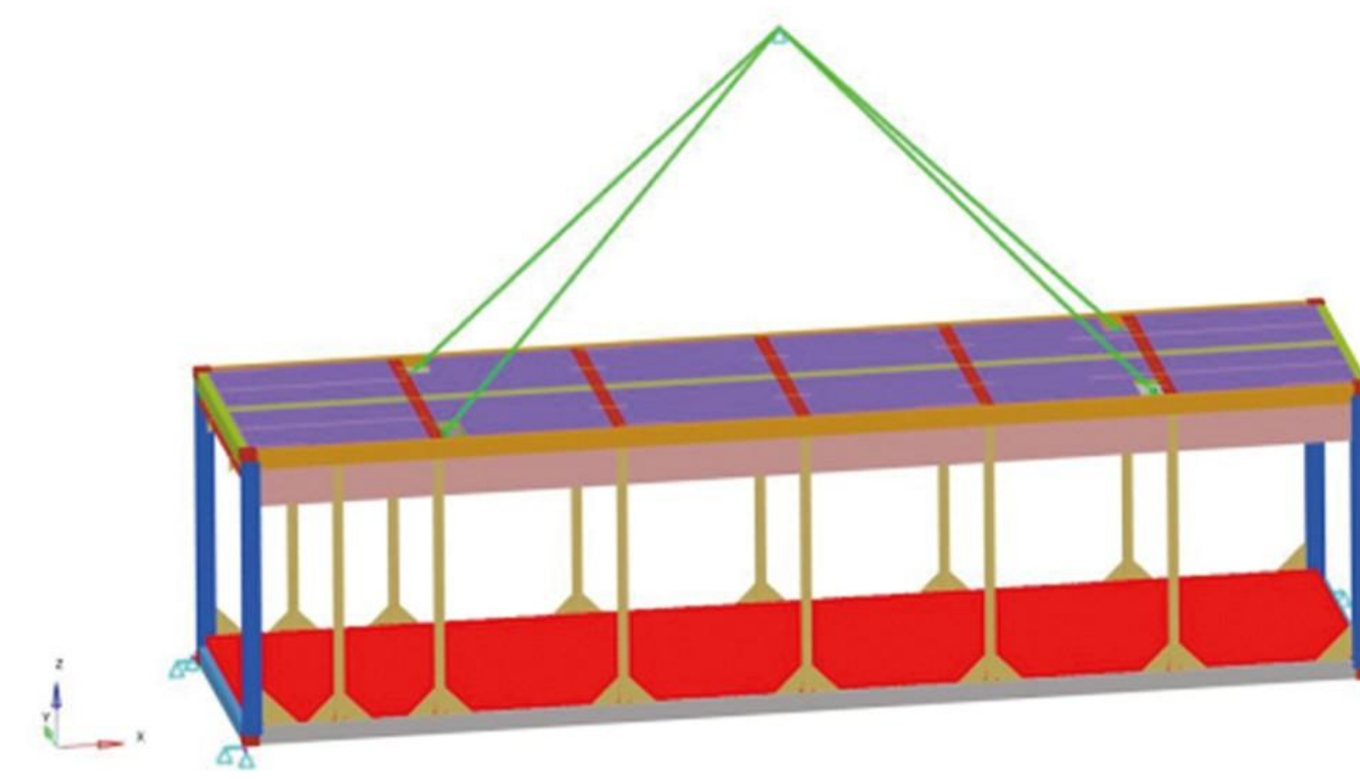
四点吊等效应力云图
