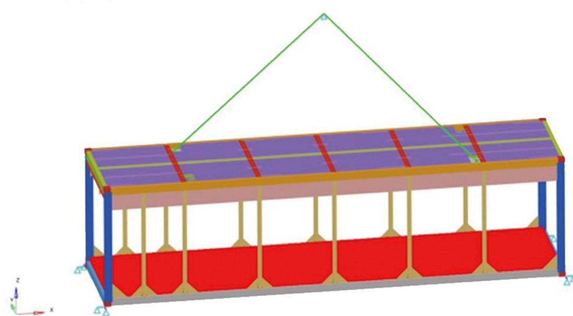
两点吊边界条件
