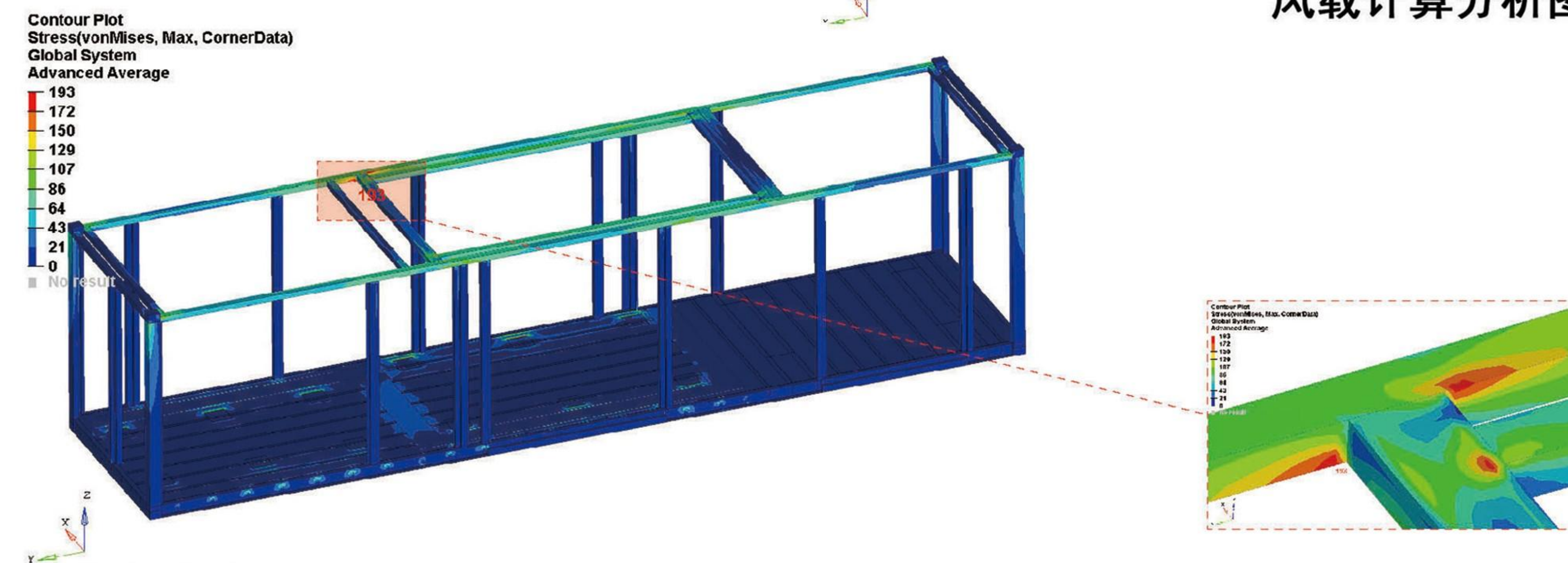
集装箱等效应力分
