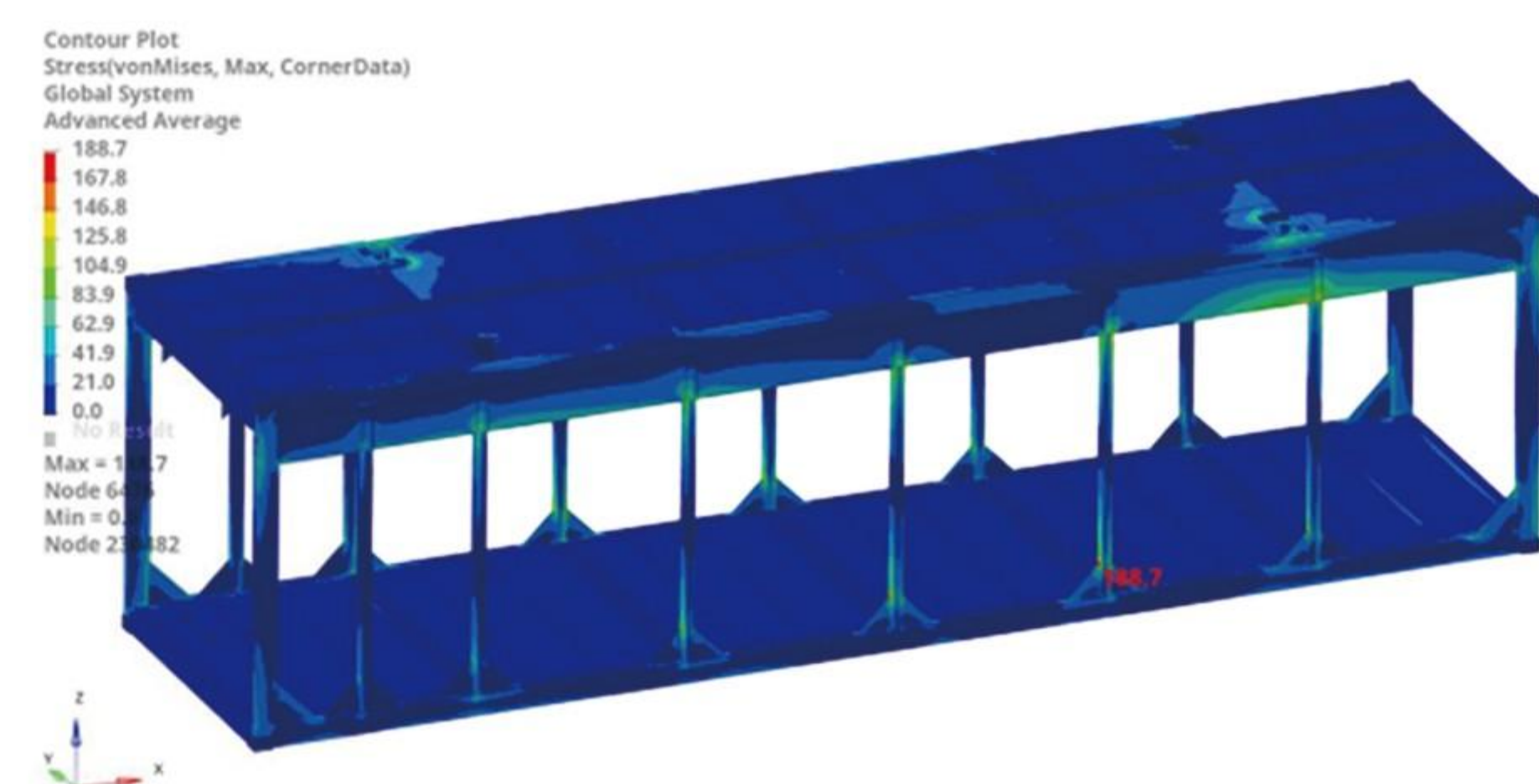
两点吊等效应力云图
