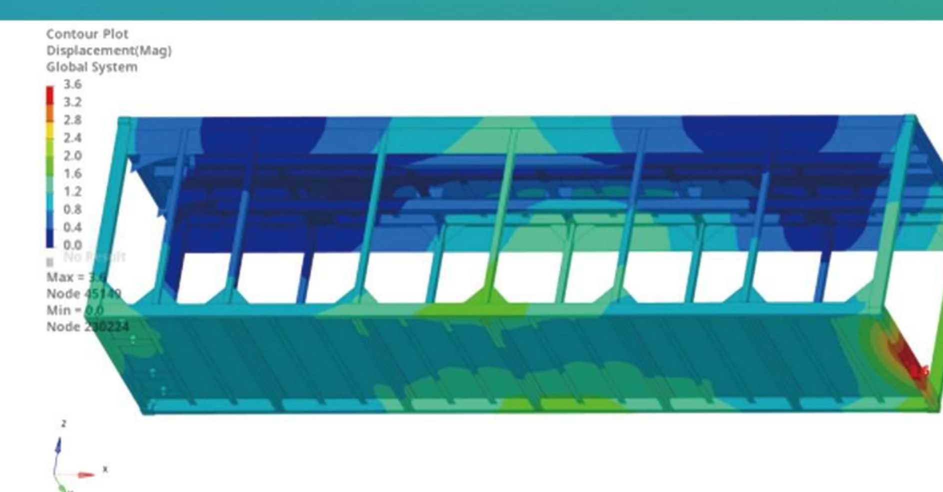
垂直冲击变形云图
