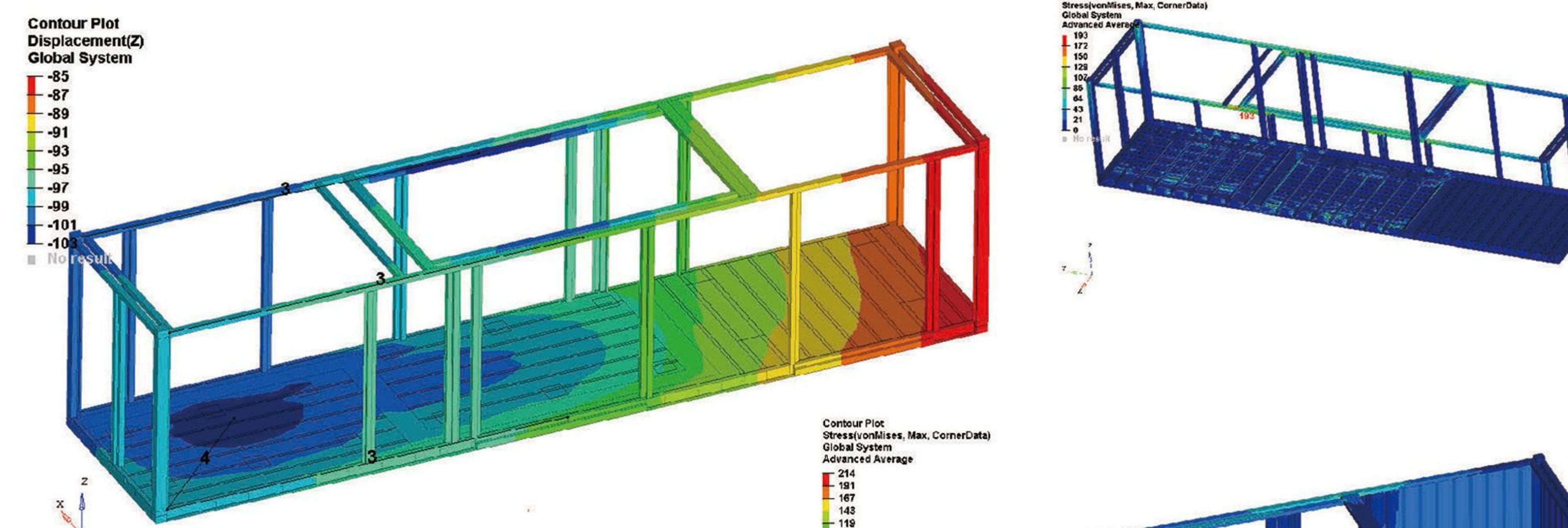
集装箱变形云图
